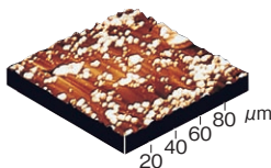
セフィオンテクトの陶器表面 100年後相当表面 (100年使用相当の加速試験結果)
