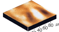
セフィオンテクトの陶器表面 100年後相当表面 (100年使用相当の加速試験結果)
